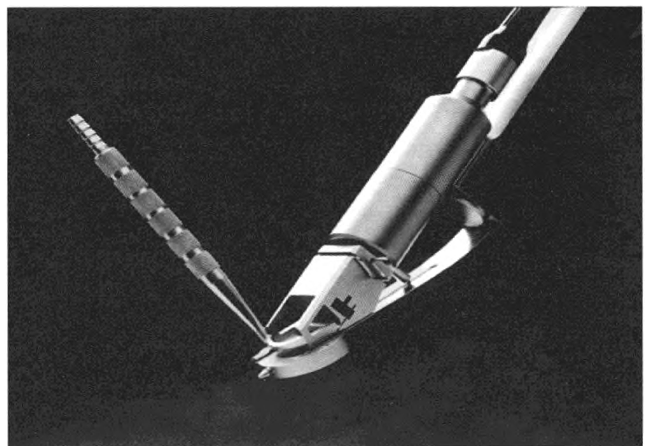
Σχήμα 3: Μικροκερατόμος
